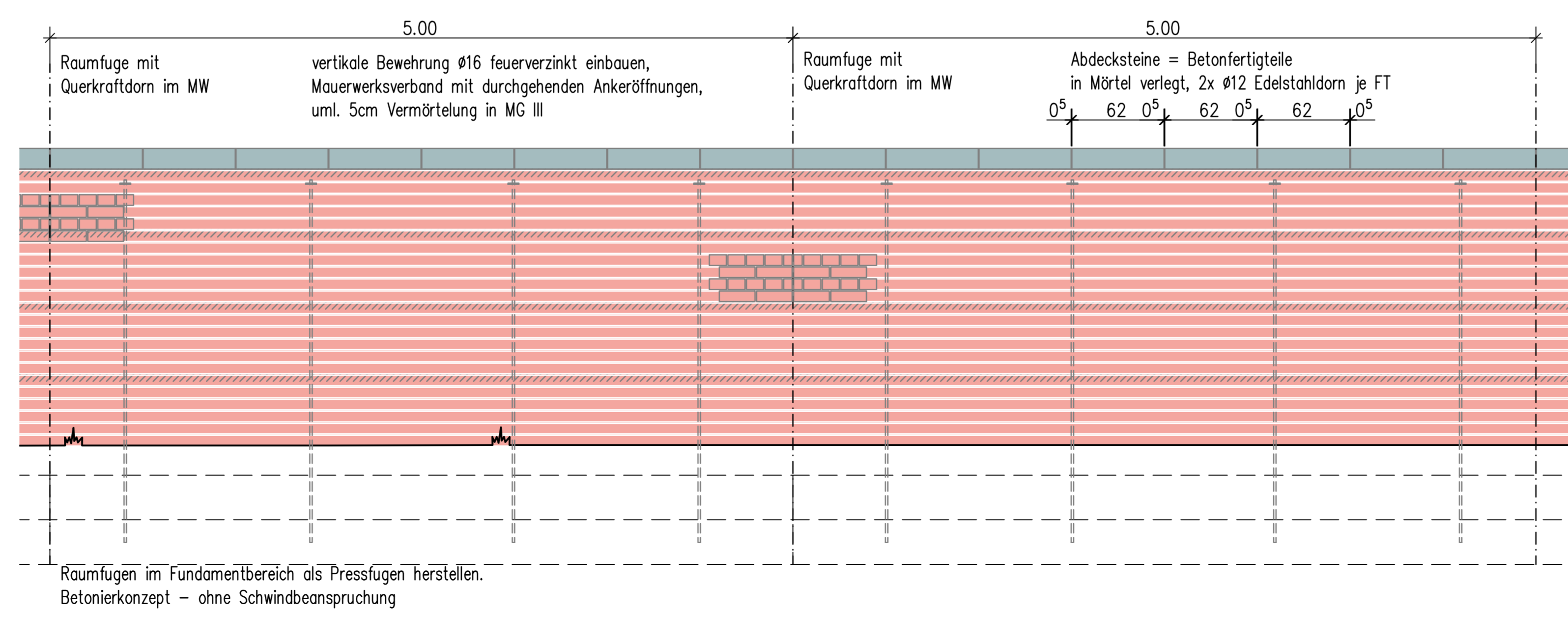
Ansicht Seite Friedhof M 1:25
