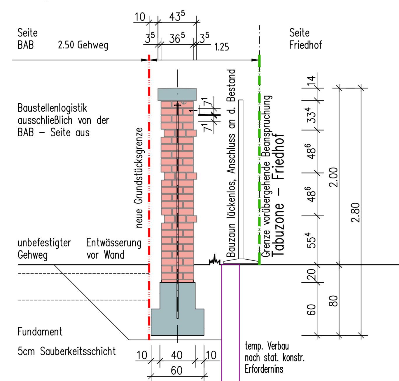
Regelschnitt M 1:25
